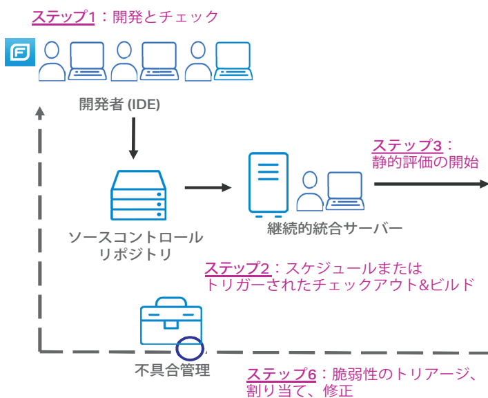
図 2 Fortify on Demand の静的アプリケーションセキュリティテストのプロセス
